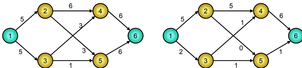
Hình 77: Mạng với các khả năng thông qua (1 phát, 6 thu) và một luồng của nó với giá trị 7
