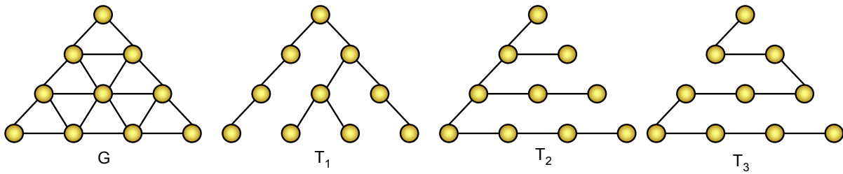
Hình 67: Đồ thị G và một số ví dụ cây khung T1, T2, T3 của nó
