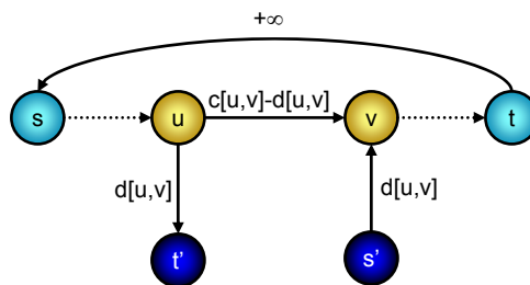
Hình 83: Mạng giả của mạng có khả năng thông qua của các cung bị chặn hai phía
