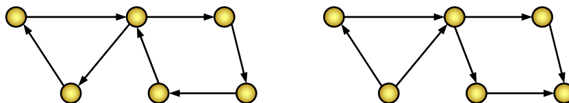
Hình 61: Liên thông mạnh và liên thông yếu
