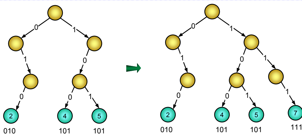
Hình 46: Với độ dài dãy bit z = 3 , cây tìm kiếm cơ sở gồm các khoá 2, 4, 5 và sau khi thêm giá trị 7
