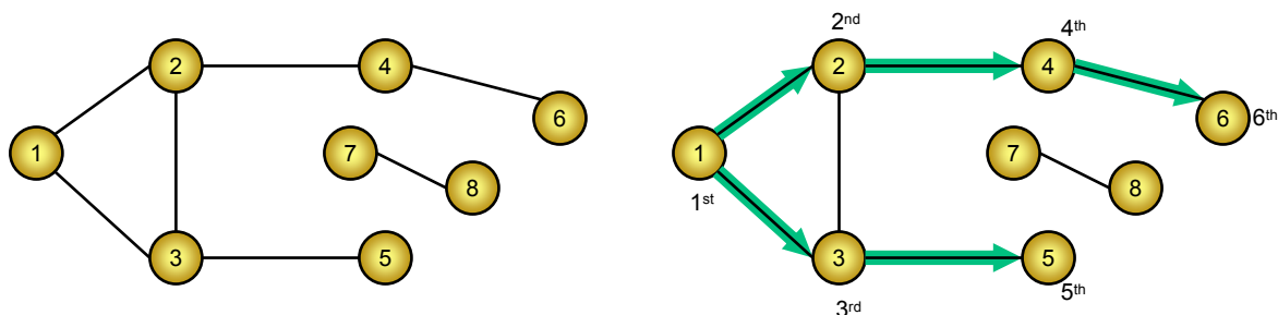
Hình 58: Cây BFS
