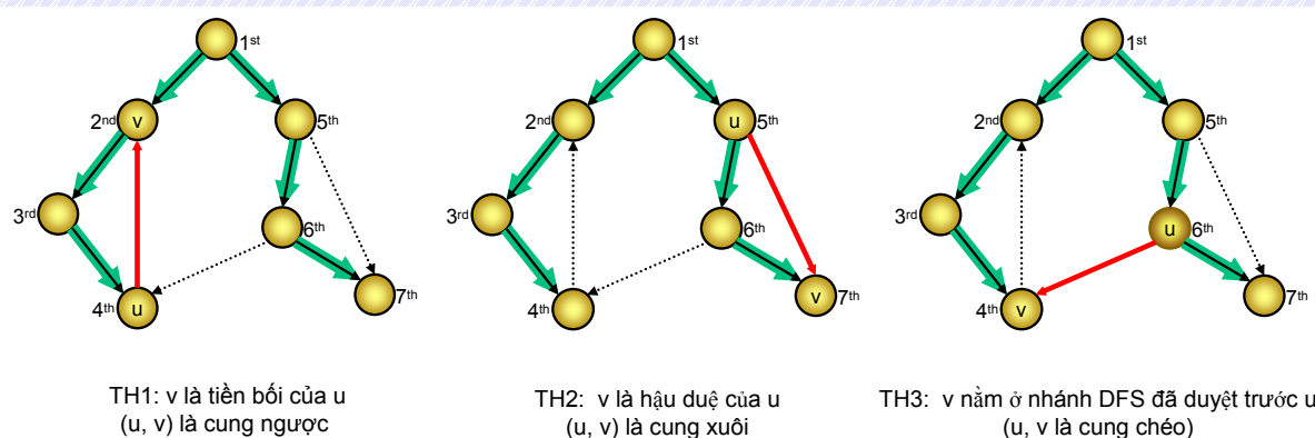
Hình 64: Ba dạng cung ngoài cây DFS
