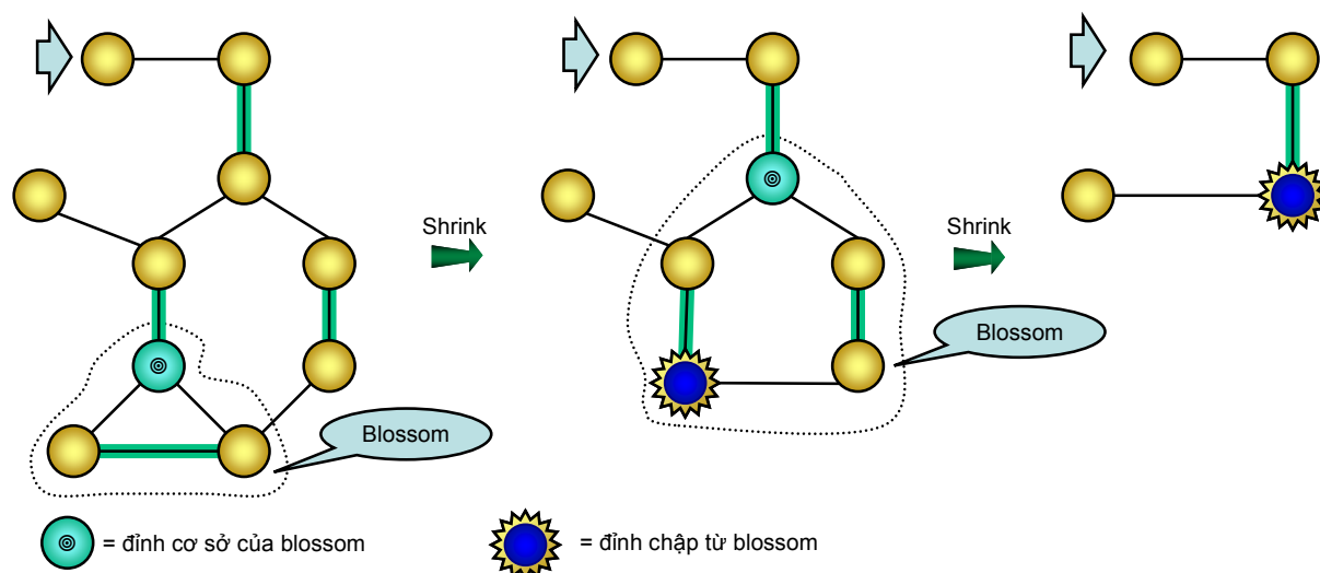
Hình 91: Phép chấp Blossom
